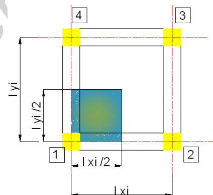
Figure 7 Vue en plan module type en
