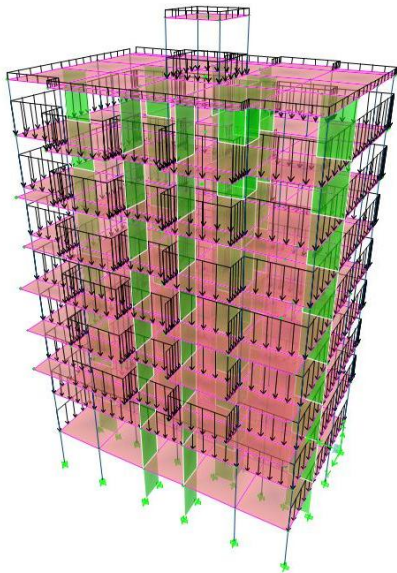
Figure 2 'vue structure tridimensionnelle 'chargée'
