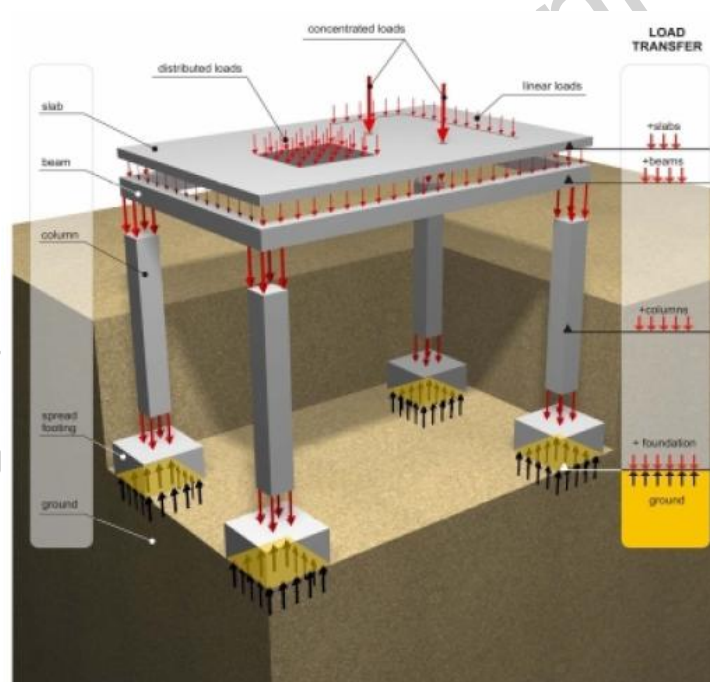
Figure 1 cheminement des efforts dans une structure
